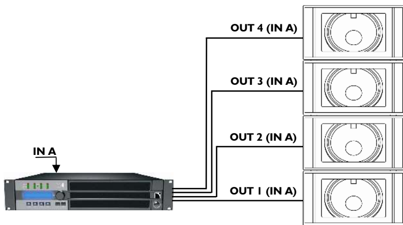
Figure 8 : Quatre SBI 18 connectés à un LA4 (configuration mono)
