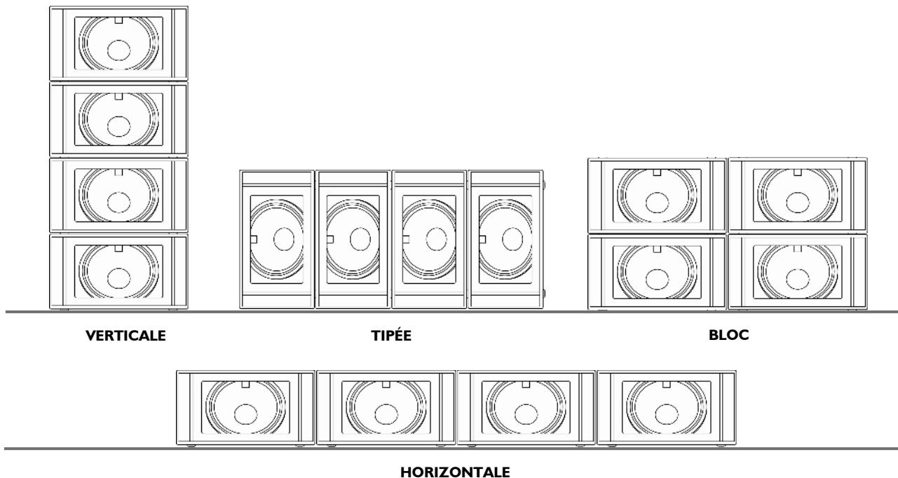
Figure 6 : Lignes SBI 18 standard basiques
