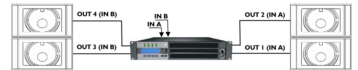
Figure 7 : Quatre SBI 18 connectés à un LA4 (configuration stéréo)
