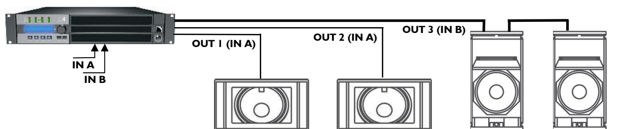
Figure 13 : Deux SBI 18 et deux ARCS® raccordés à un contrôleur LA4
