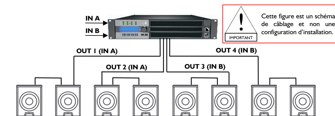
Figure 5 : 8 enceintes 8XTi connectées à un contrôleur LA4 / LA4X
