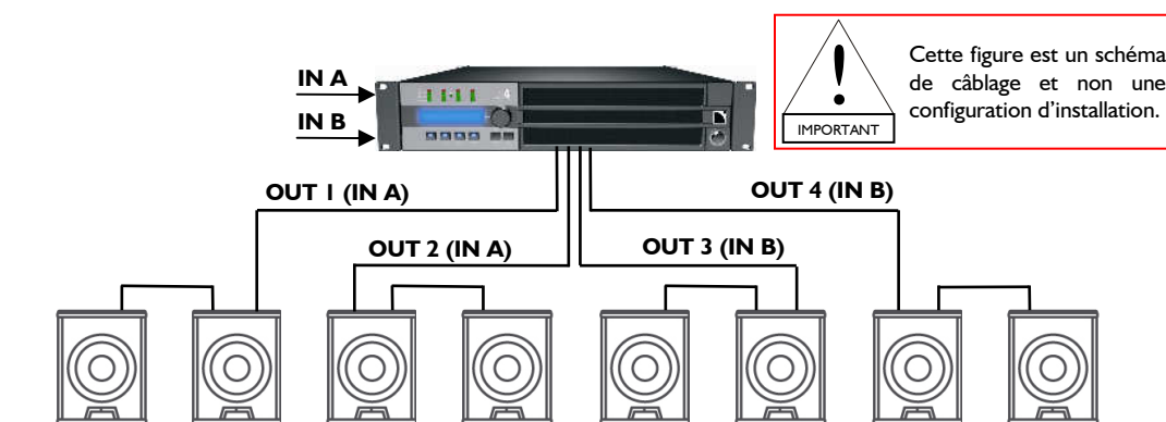
Figure 4 : Huit enceintes 8XTi connectées à un contrôleur LA4 / LA4X
