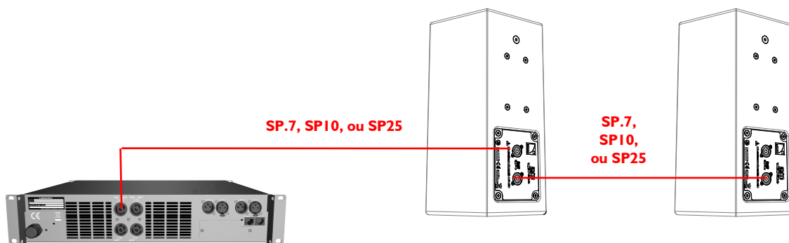
Figure 3 : Raccordement de deux 8XTi en parallèle sur le canal I du LA4 / LA4X
