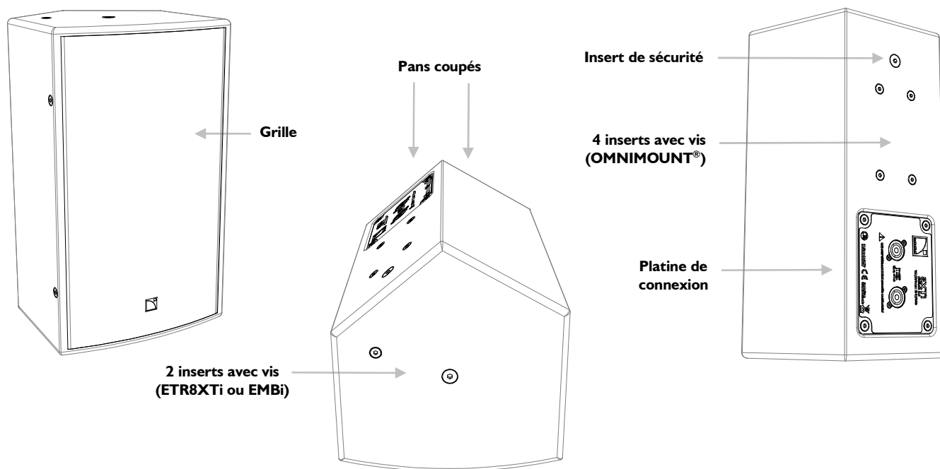
Figure 2 : L'enceinte 8XTi
