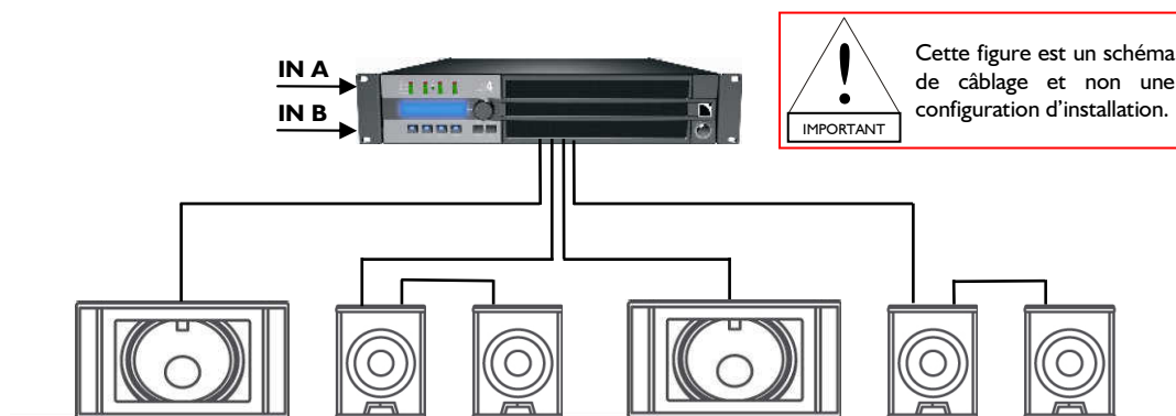
Figure 6 : Quatre 8XTi et deux SB18i connectées à un contrôleur amplifié LA4 / LA4X
